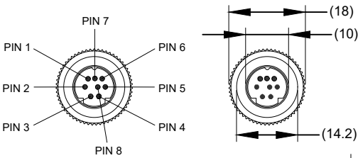
8 PIN MINI DIN FEMALE MATING FACE
